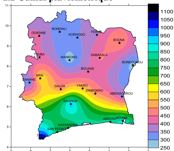
Fig 3: Cumul pluviométrique (mm) du 1 janvier au 30 Juin 2016
