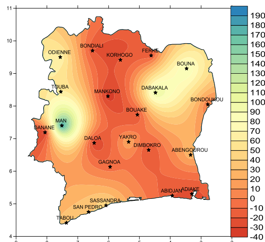
Fig 9: Bilan hydrique climatique (mm) du 21 au 30 Juin 2016
