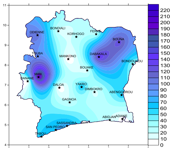
Fig1: Pluviométrie totale (mm) du 21 au 30 Juin 2016
