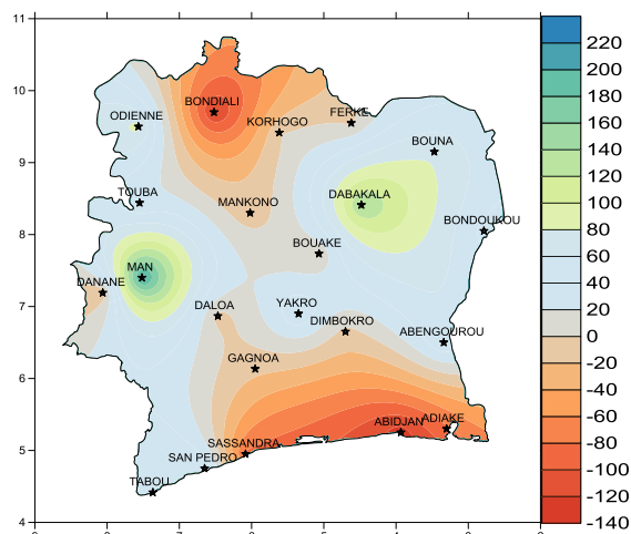
Fig2 : Ecart entre la pluviométrie (mm) du 21 au 30 Juin 2016 et du 21 au 30 Juin 2015
