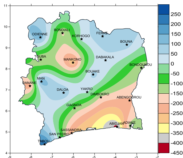
Fig 4 : Ecart entre Cumuls pluviométriques du 1 janvier au 30 Juin 2016 et du 1 janvier au 30 Juin 2015
