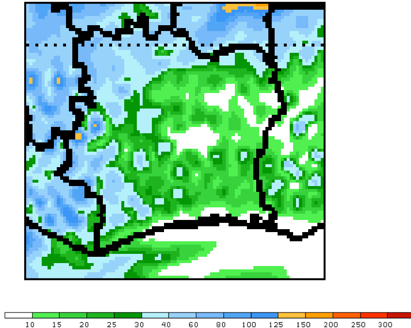
Figure 10 : prévision de la pluviométrie du 04 au 11 Juillet 2016 (source : NOAA, climate Prédiction Center)
