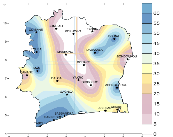
Fig 08: Réserve en eau des sols (mm) de RU= 60 mm
